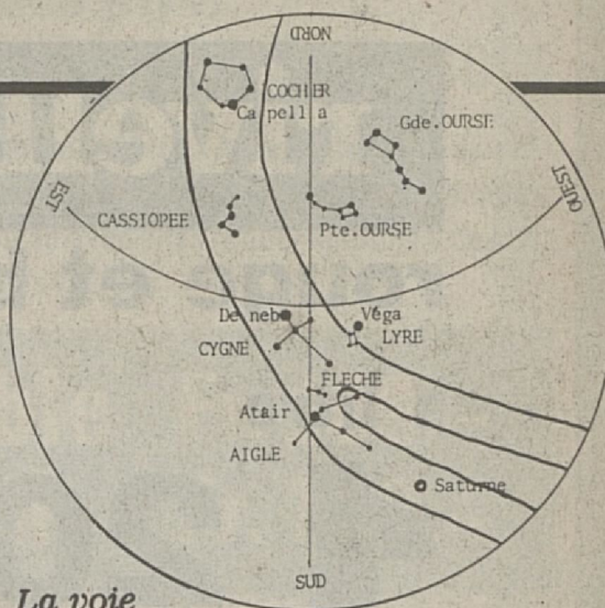
La voie lactée à la mi-septembre, à 22 h.
